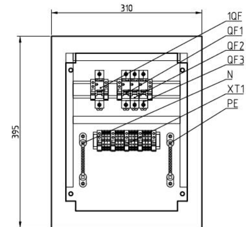
Рисунок 3.1 Компоновка изделия.
