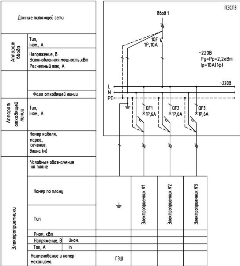
Рисунок 4.2 Схема линейная.
