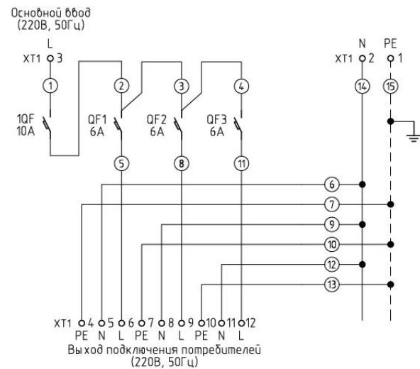
Рисунок 4.1 Схема подключения.
