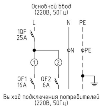
Рисунок 4.1 Схема подключения.
