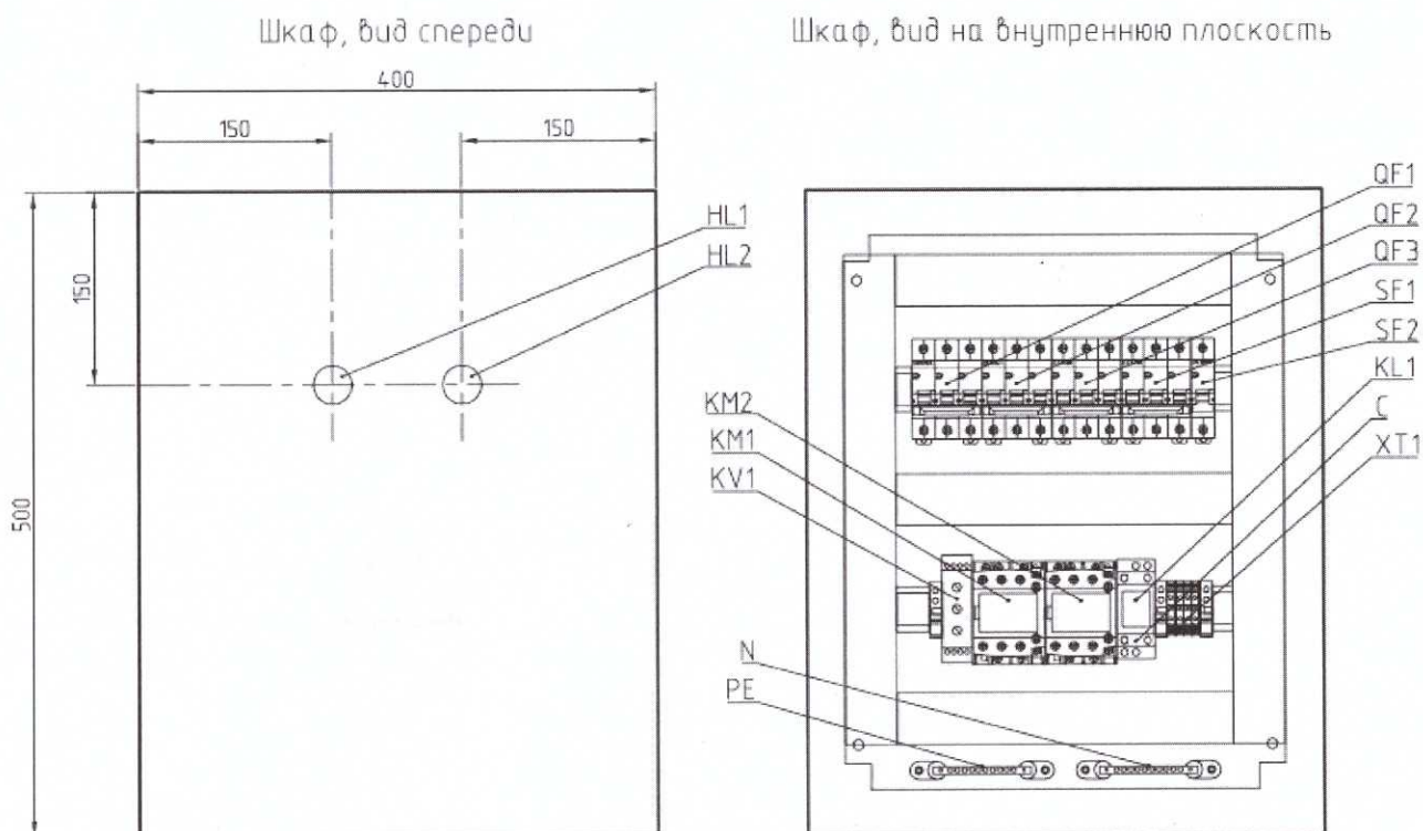
Рисунок 3.1 Компоновка и внешний вид шкафа.
