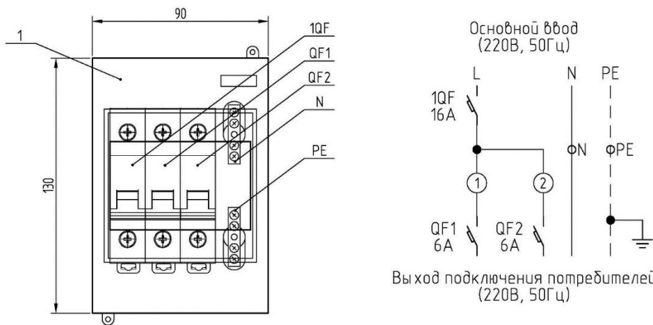
Рисунок 3.1 Компонировка изделия и схема подключения.
